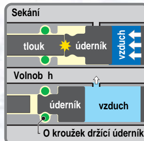
Zádný přiklep při volnobě Zajišťuje delší životnost stroje
