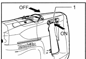
1. Přepínací páčka
